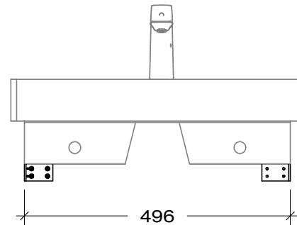
2. ติดตั้งเหล็กฉาก
