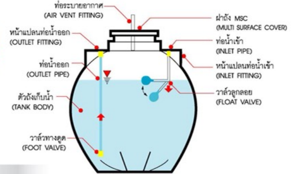
รุ่น 3000-6000 ลิตร (รุ่นฯ NET-TECH)
