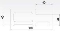
Section วงกบ WPC 2"x4"
