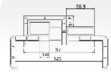
Section วงกบ UPVC Subframe H
