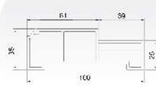
Section วงกบ UPVC 2"x4"
